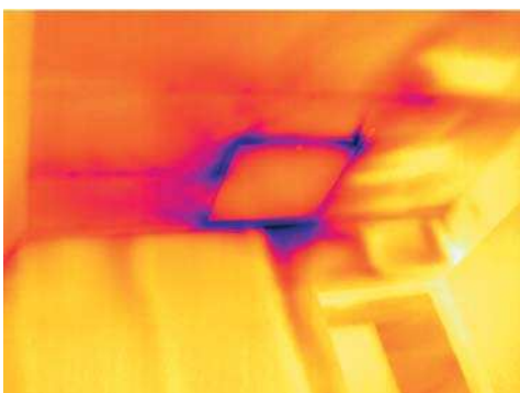
Error de instalación. La puerta de acceso no sella correctamente. Observe que el termograma también muestra la presencia de fallos de aislamiento.
