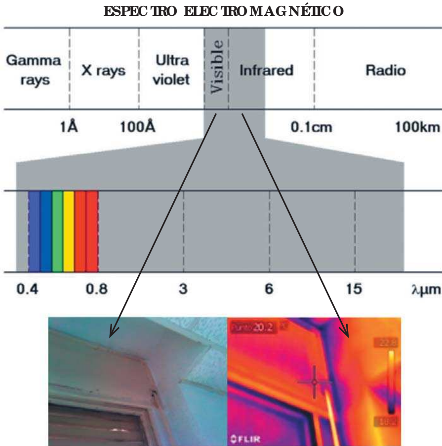
Figura 3. Espectro electromagnético.
