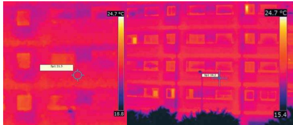
Figura 9. Imágenes infrarrojas de una fachada.
