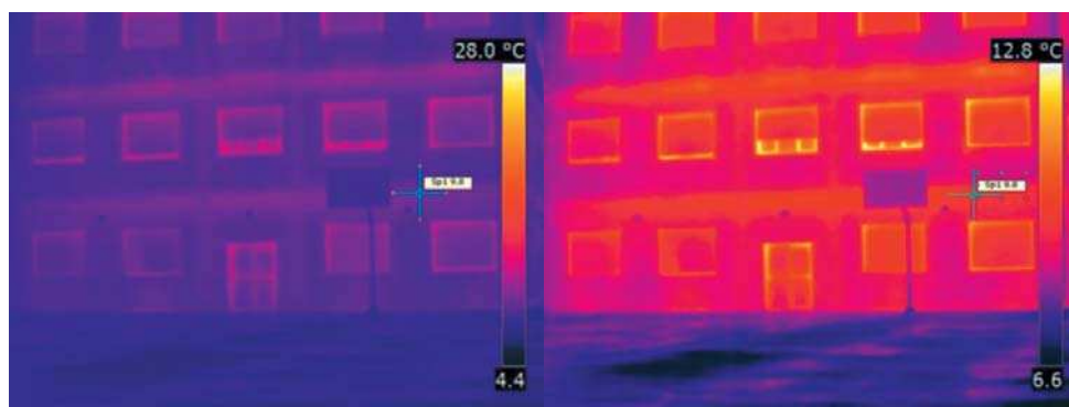
Figura 11. Una misma imagen infrarroja, con el mismo rango pero con distinto campo.
