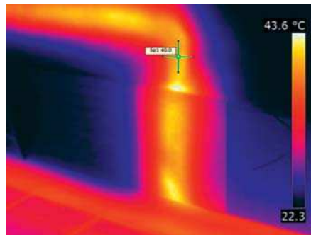
Figura 1. Imagen infrarroja de la acometida a un colector de suelo radiante.
