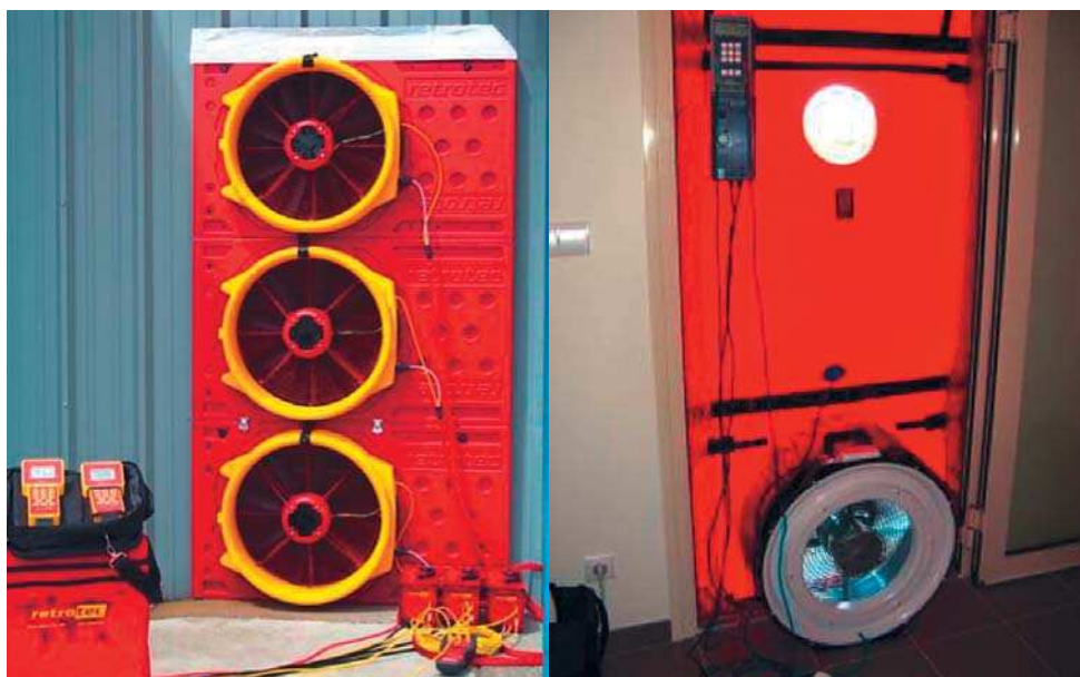
Fotografías 1 y 2. Ejemplos de equipos de infiltrometría manufacturados por los fabricantes más reconocidos.
